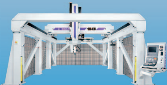
Portalfräsmaschine JP Gantry Standard 5m x 2,5m x 1m
