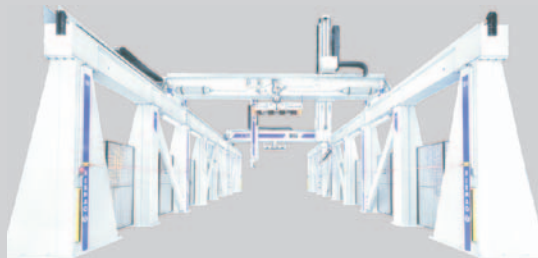
Doppelportale und Sonderlösungen bis 60m x 12m x 8,5m
