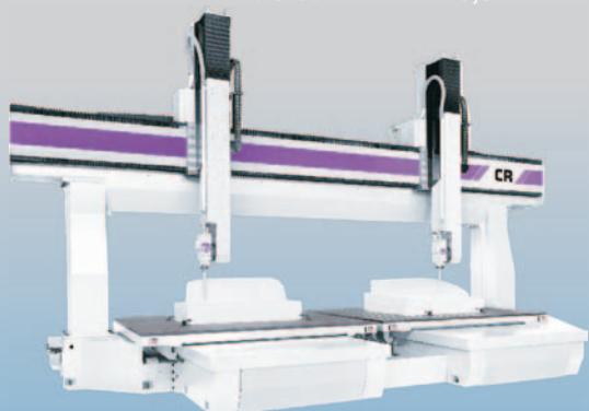
CR Twin Standard 2x (3m x 3m x 1m) oder gekoppelt 1x (6m x 3m x 1m)
